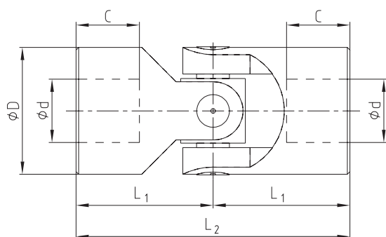
Präzisions-Einfachgelenk X
