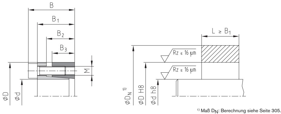
Anwendungsbeispiel Nabenform
