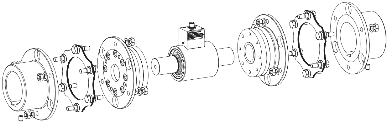
DATAFLEX® 42
