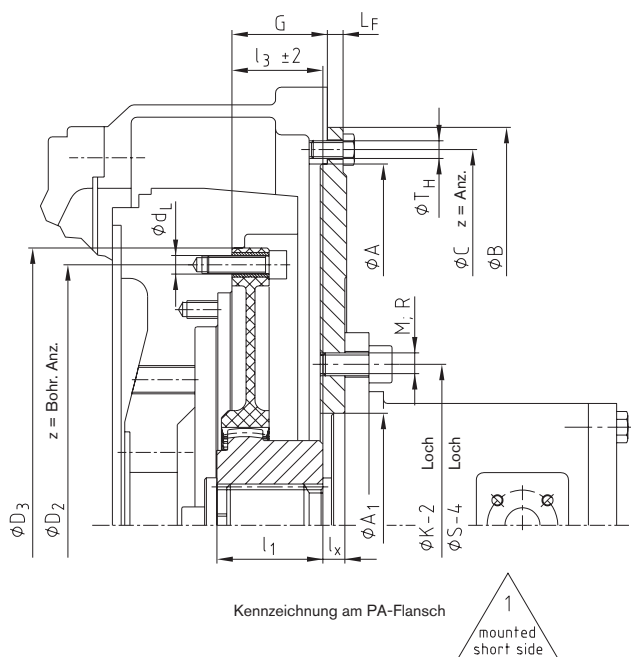
Kupplungseinbau kurz ( l_3 )
