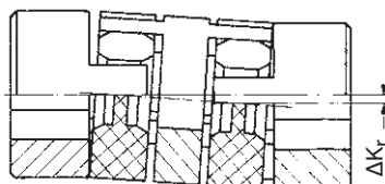
Radialverlagerung
