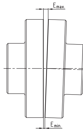
Winkelverlagerung \Delta K_w
