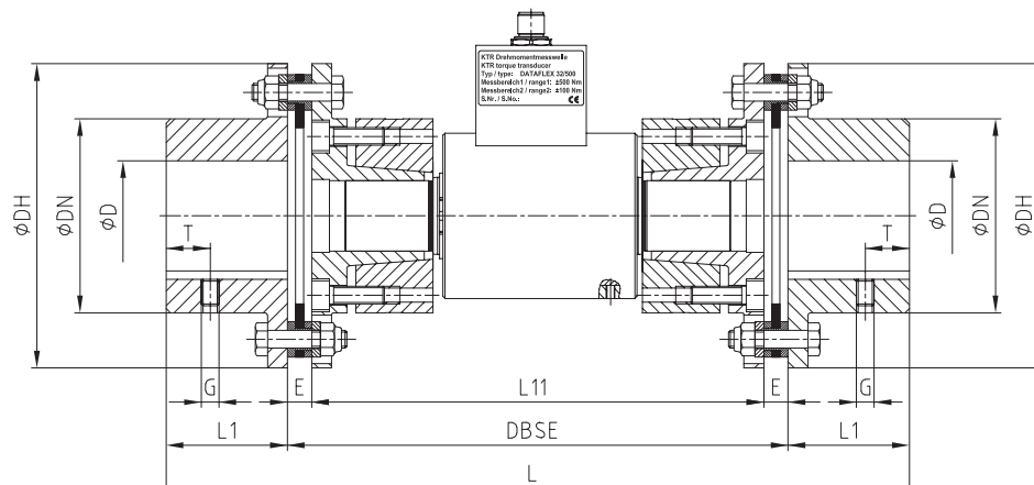
Abmessungen [mm] der Drehmomentmesswelle und der Kombination mit RADEX®-NC HT Kupplungen
