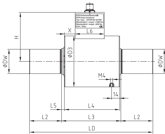
DATAFLEX® 42
