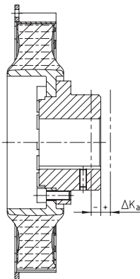
Axialverlagerung
