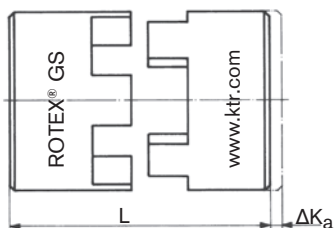
Axialverlagerung
