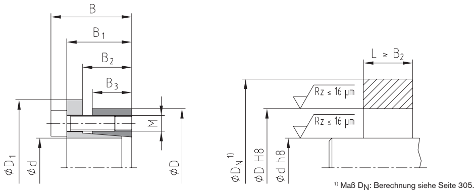
Anwendungsbeispiel Nabenform
