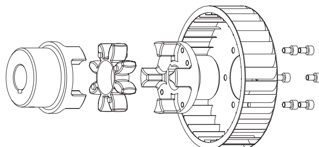
Bauart FNN mit Lüfter (Type 1)
