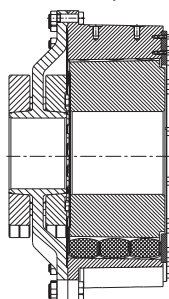
Bauart AFN mit Spannringnabe
