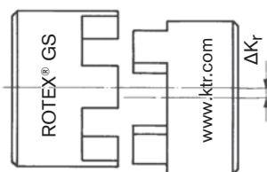
Radialverlagerung
