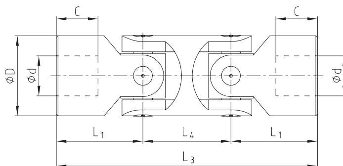
Präzisions-Doppelgelenk GD
