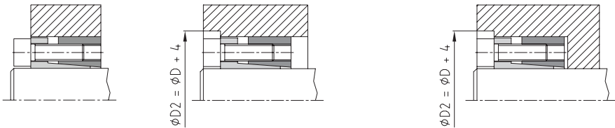
Anwendungsbeispiel Nabenform
