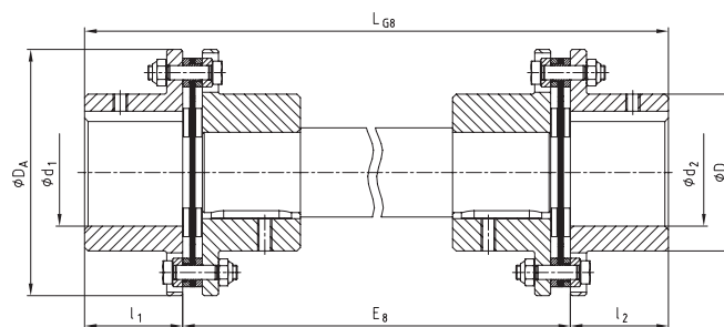
Bauart NNW
