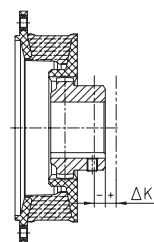
Axialversatz \Delta K_a
