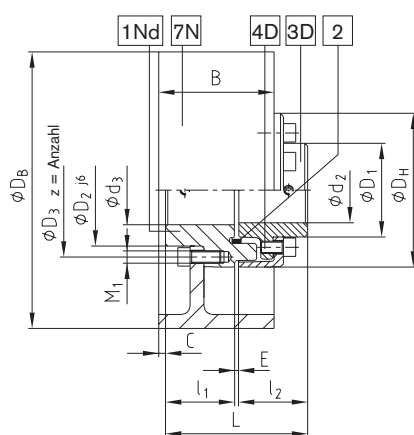
Bremsstrommel Bauart ADR-BTA
