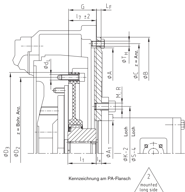
Kupplungseinbau lang ( l_7 )
