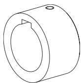
Ausf. 1.0 mit Passfedernut und Gewindestift
