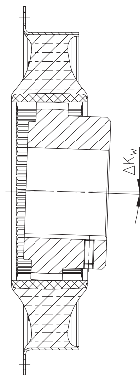
Winkelverlagerung
