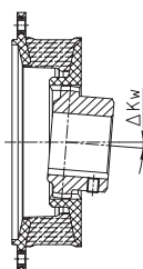
Winkelversatz \Delta K_w
