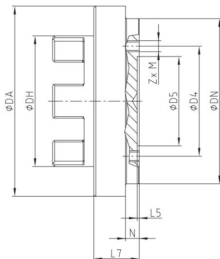
Abmessungen [mm]
