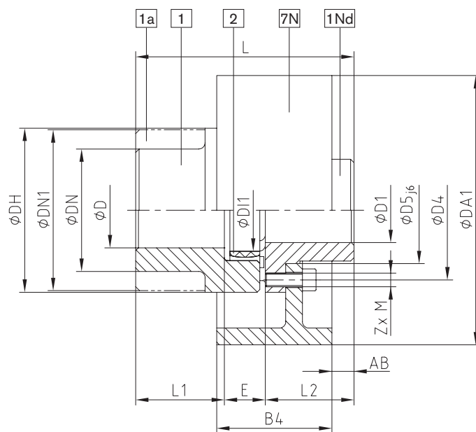
Bremstrommel Bauart BTAN
