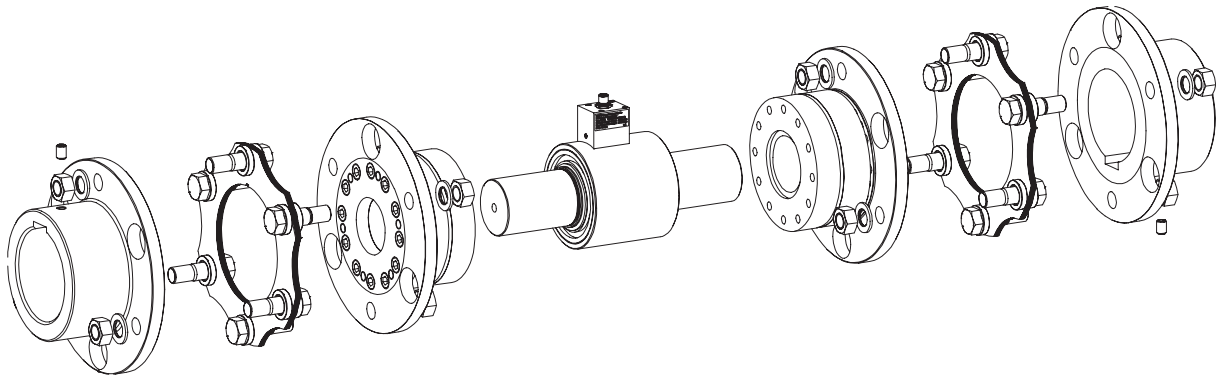
DATAFLEX® 70
