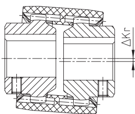
Verlagerungen – Bauart junior Kupplungen
