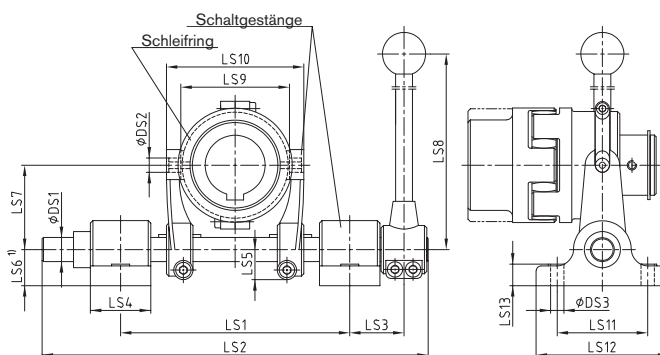
Bauart SD mit Schleifring und Schaltgestänge
