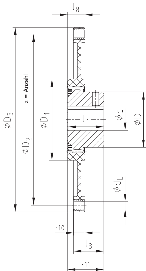
Anbau kurz
