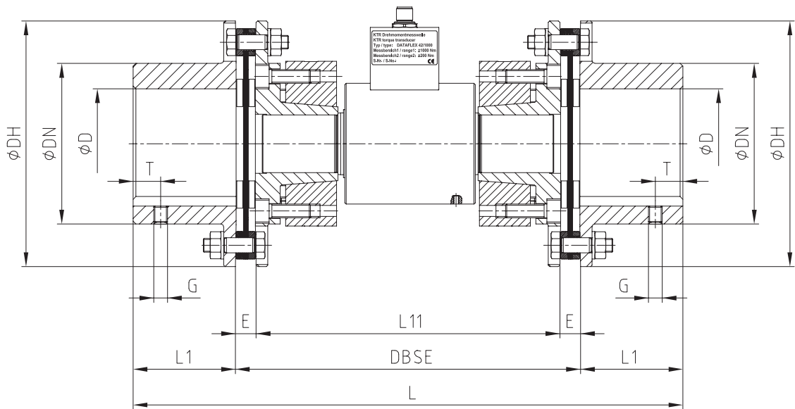
Kombination DATAFLEX® 42 mit RADEX®-N
