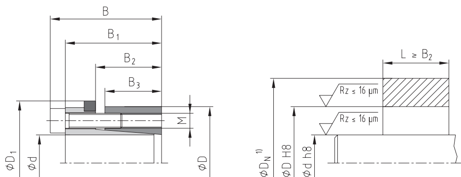
Anwendungsbeispiel Nabenform
