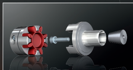
ROTEX® GS Spreiznabe
