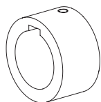
Ausf. 1.0 mit Passfedernut und Gewindestift
