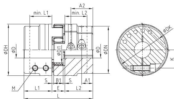
ROTEX® 38 - 90
