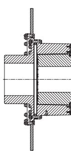
Bauart AFN mit Bremsscheibe
