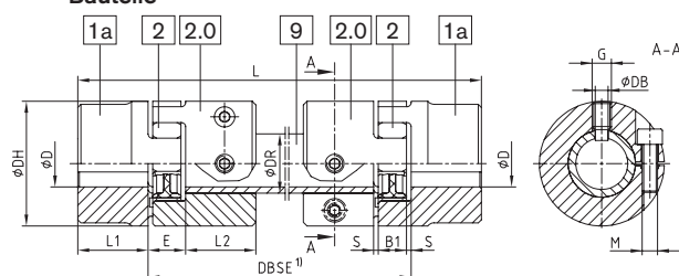
Bauart ZR (mit GS-Zahnkranz) 3)
