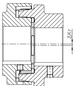
Radialverlagerung ΔK r
