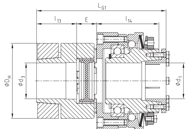
Nabenausführung 6.0
