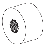
Ausf. 1.3 Profilverzahnung
