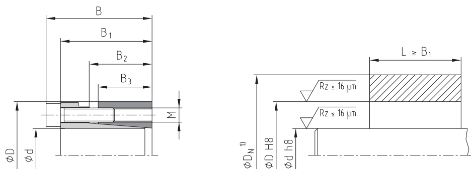
Anwendungsbeispiel Nabenform
